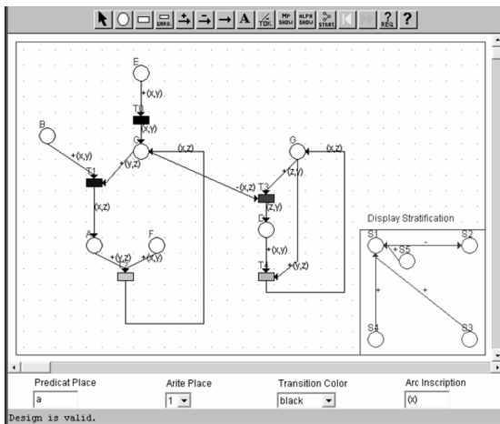
Fig. 5. STRPRO Debugger
