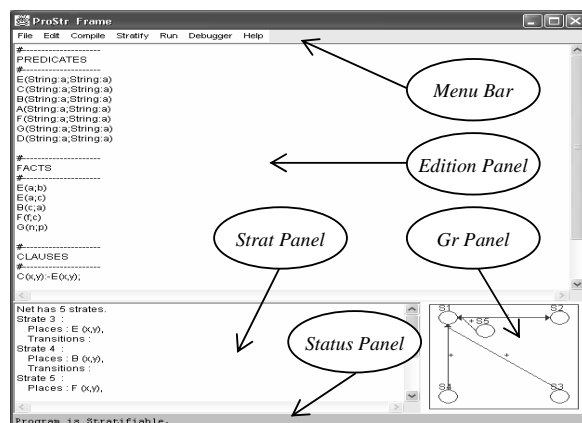
Fig. 4. STRPRO interface
