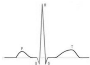
Fig. 3 Heart Wave
