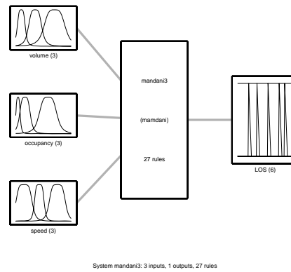
Fig. 6. Mamdani FIS
