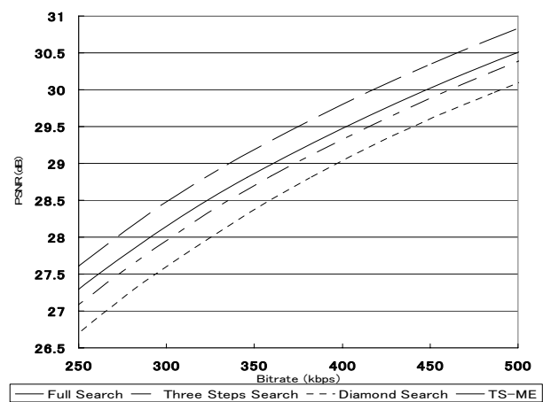
Fig. 21 PSNR-Bus
