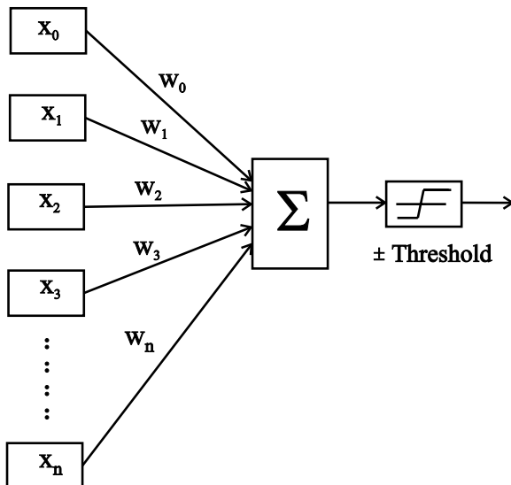
Fig. 2 Perceptron
