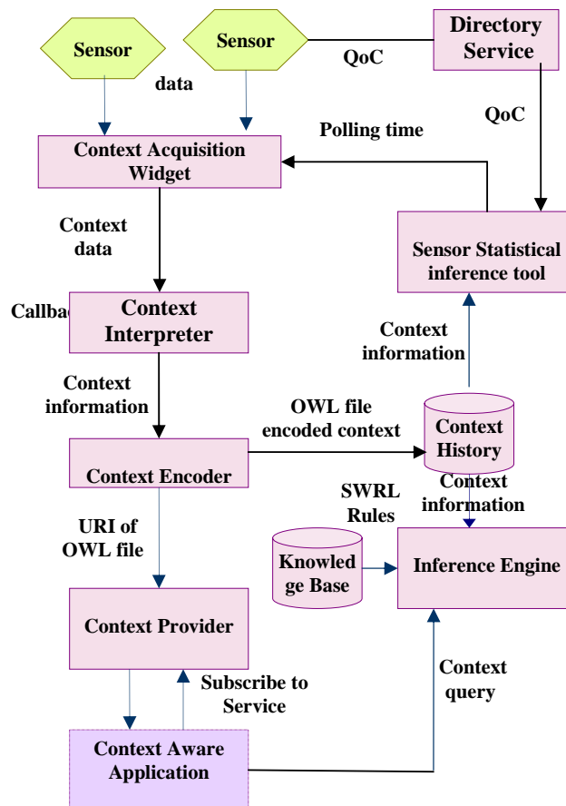
Fig. 2 Module interaction
