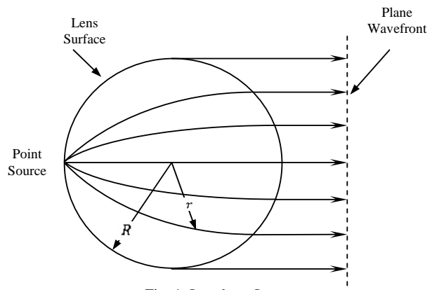
Fig. 1: Luneburg Lens
