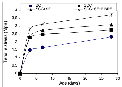
Fig. 2 Tensile stress
