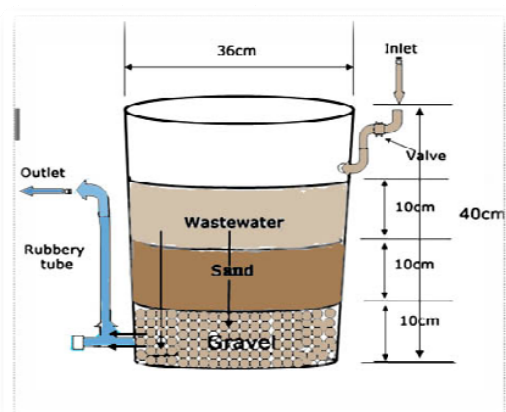
Fig. 3 Sand Filtration Pot
