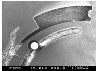
Fig. 2 PDMS mold
