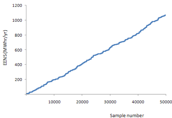
Fig. 1 Accumulation characteristics of EENS for RBTS system
