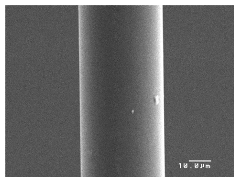
PA6-5000 m/min
