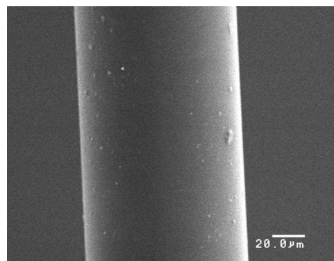
PA6-500 m/min
