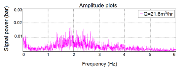
(d) Amplitude plots for Q=21.6 m 3 /hr
