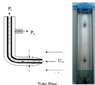
Fig. 6 Pitot tube
