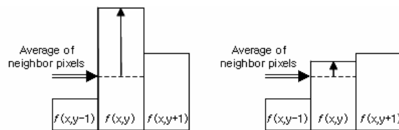
Fig. 3 Blur estimation
