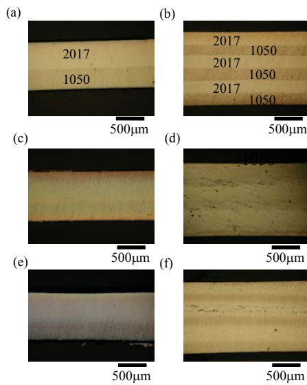
Fig. 3 OM images of 2- and 6-layered clad structures, (a) 2LAR, (b) 6LAR, (c) 2LHT 400, (d) 6LHT 400, (e) 2LHT500, (d) 6LHT 500
