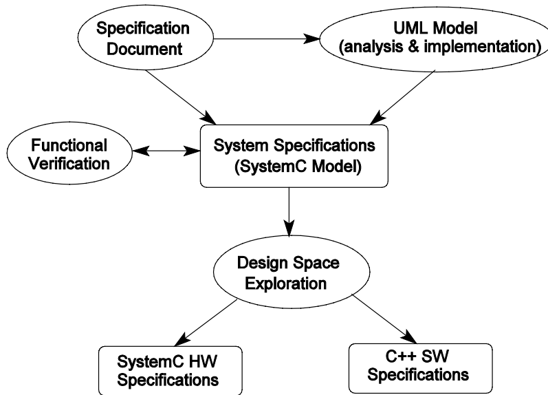
Fig. 1 UML SystemC
