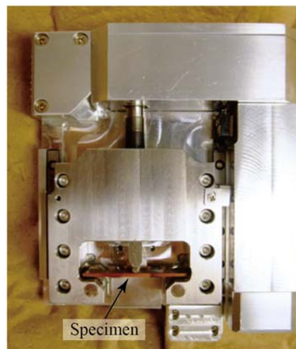
Fig. 2 Bending apparatus
