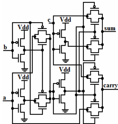
Fig. 4 TGCMOS
