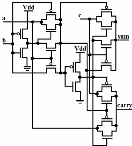
Fig. 6 TFA
