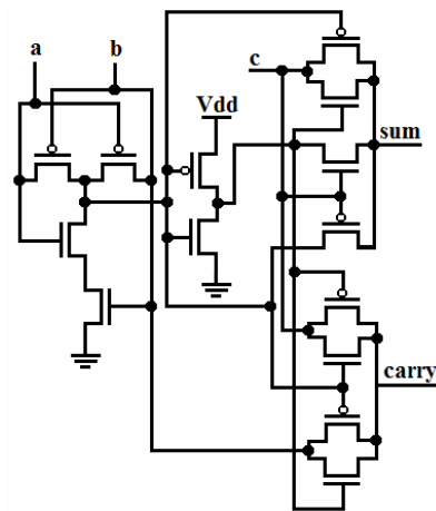
Fig. 5 14T
