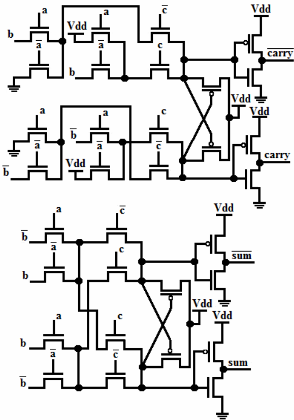
Fig. 2 CPL
