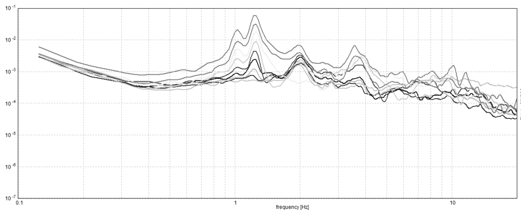
Fig. 6 Amplitude spectra
