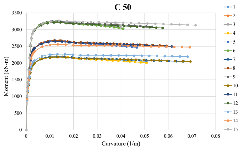
Fig. 5 (d) MC relationship for C50
