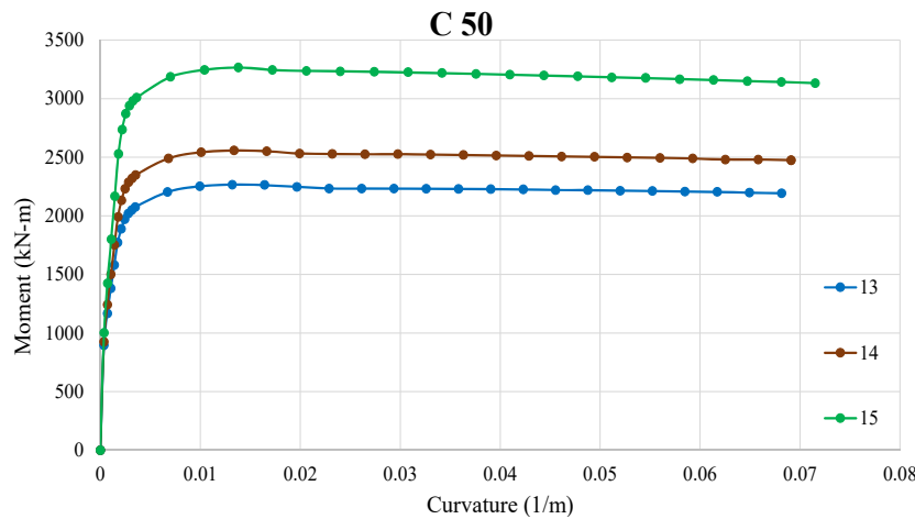
Fig. 7 (d) MC relationship with longitudinal reinforcement type
