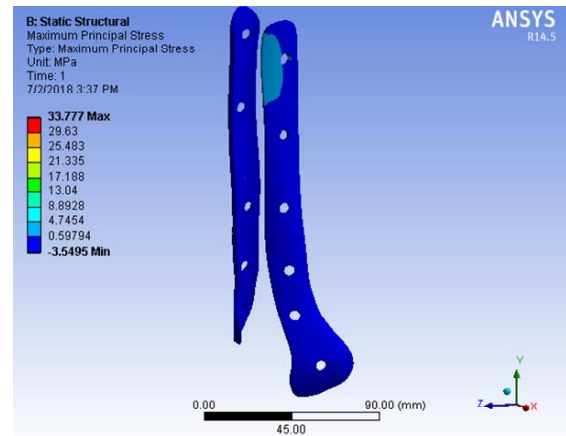
Fig. 8 (d) Maximum principal stress in implants
