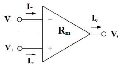
Fig. 1 Block diagram of the OTRA
