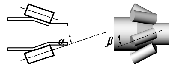
Fig. 7 Roller Angles
