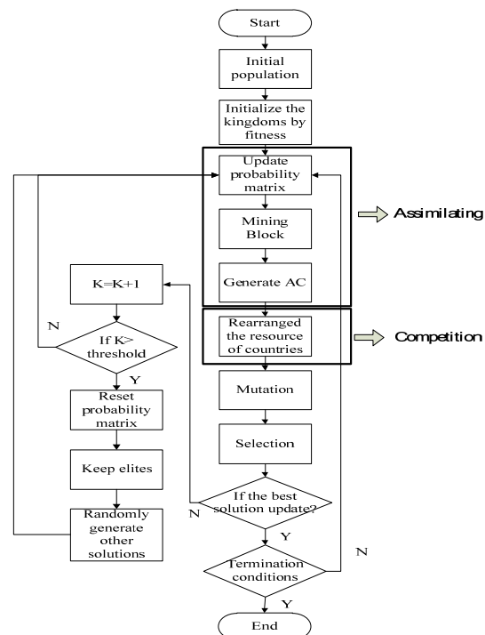
Fig. 2 BICAGS flowchart
