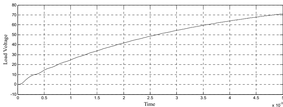
Fig. 12 Load voltage
