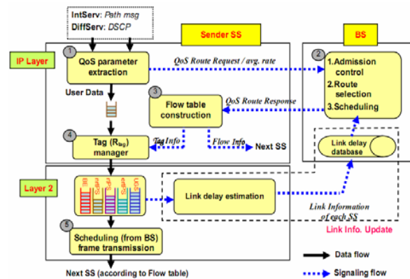
Fig. 2 QoS framework
