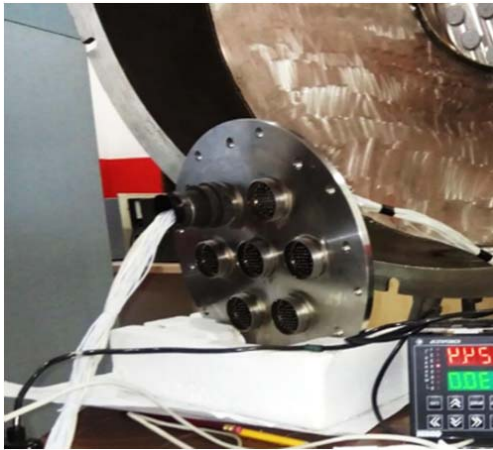
Fig. 16 MVC interface
