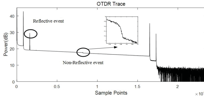
Fig. 1 OTDR trace
