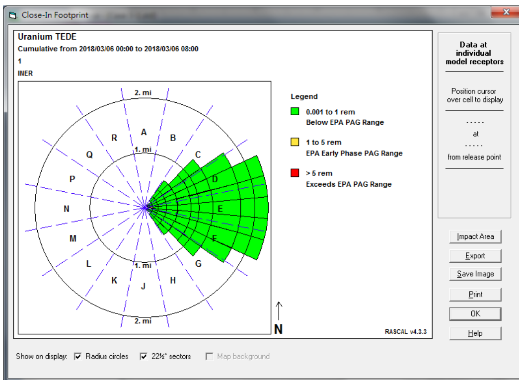
Fig. 4 The UF6 analysis result for Uranium TEDE
