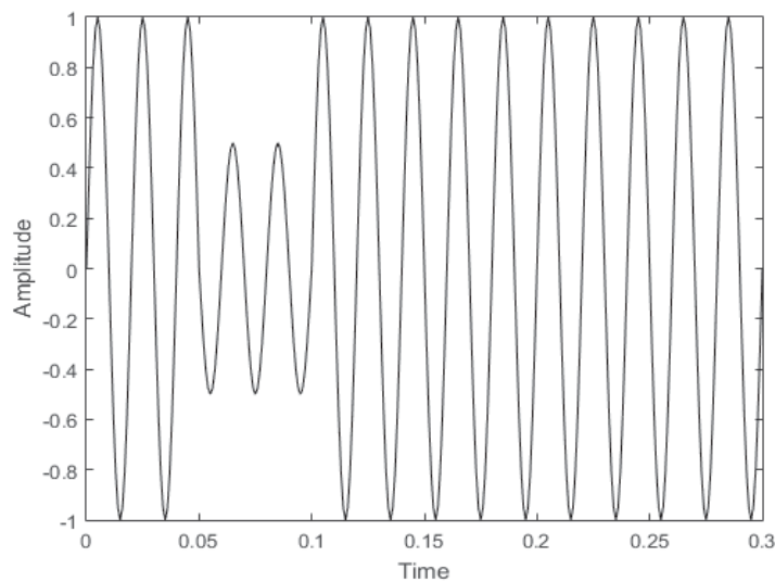
Fig. 2 Sag signal
