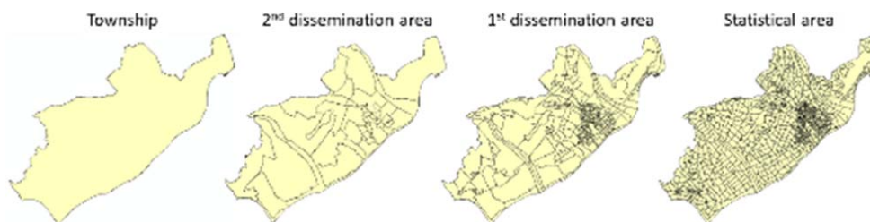
Fig. 1 TGSC framework
