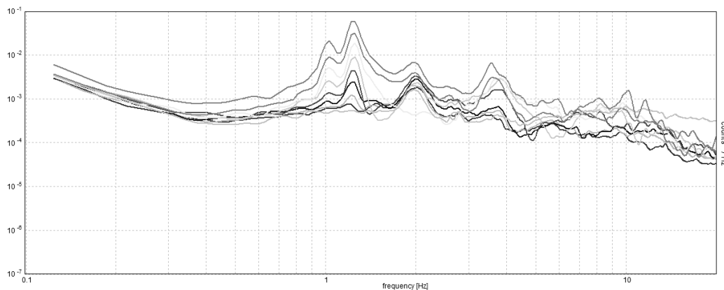
Fig. 6 Amplitude spectra
