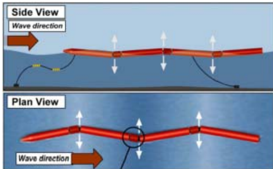
Fig. 9 Pelamis model [17]
