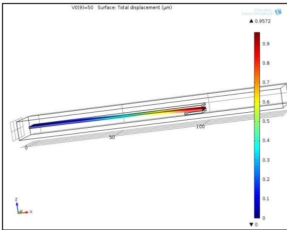
Fig. 4 Electrostatic actuator
