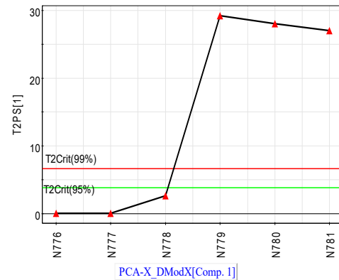
PCA-X DModX[Comp. 1]
