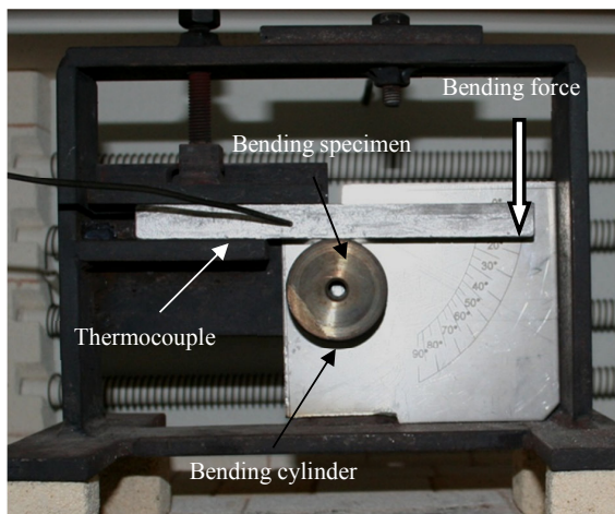
Fig. 2 Bending test apparatus
