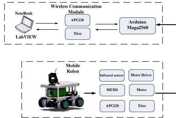
Fig. 3 Communication Module
