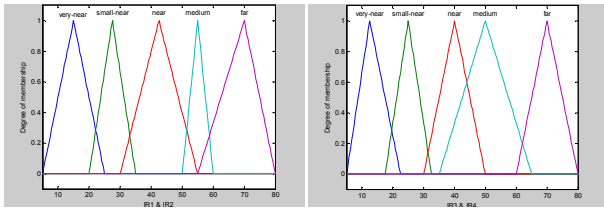
(a) (IR 1 , IR 2 ) pair MF (b) (IR 3 , IR 4 ) pair MF
