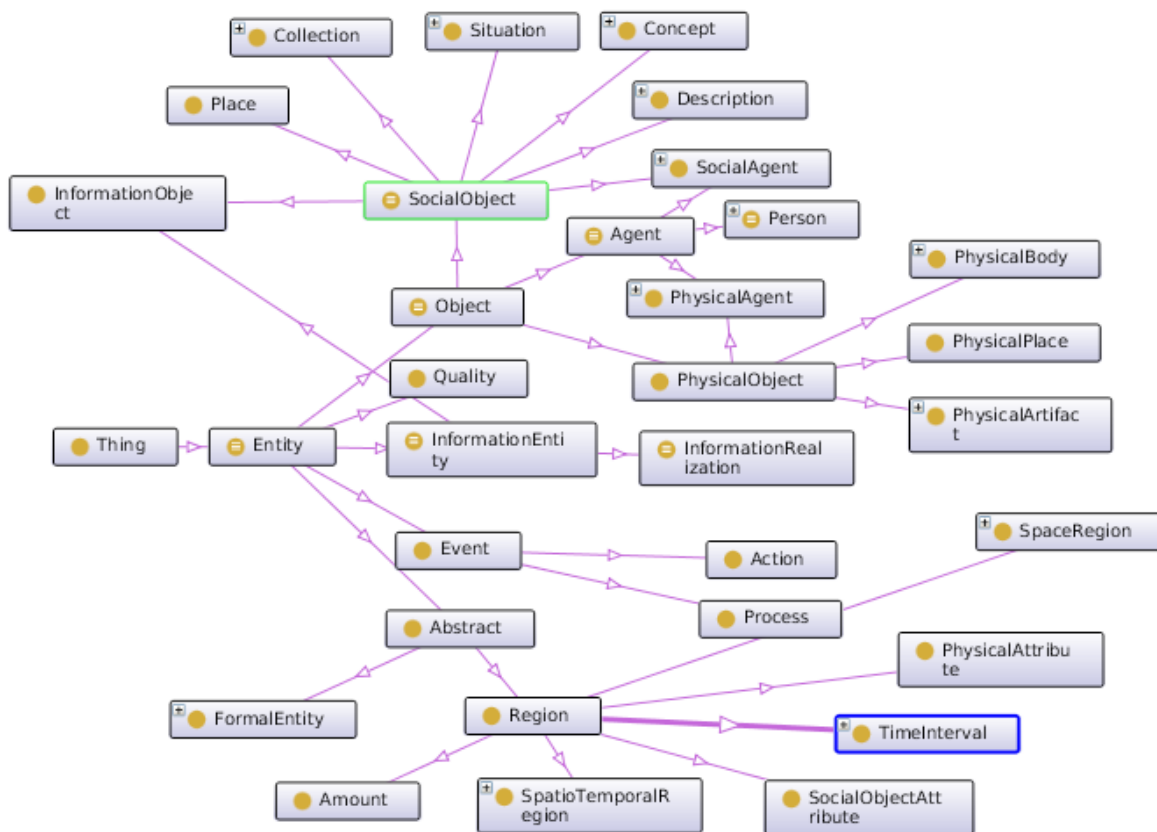
Fig. 6 Event-Model-F [6]
