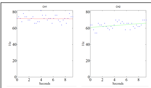
Fig. 3 MDF estimator
