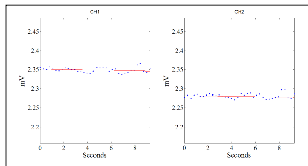
Fig. 5 RMS estimator
