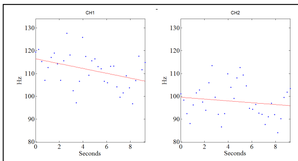
Fig. 2 MNF estimator
