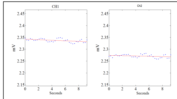
Fig. 4 ARV estimator
