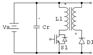
Fig. 3 Bifiller Converter
