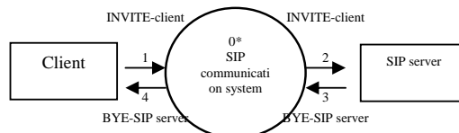
Fig. 1 DFD level 0
