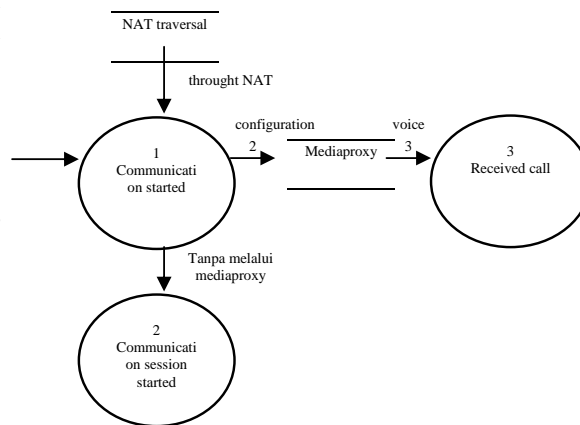
Fig. 2 DFD level 1
