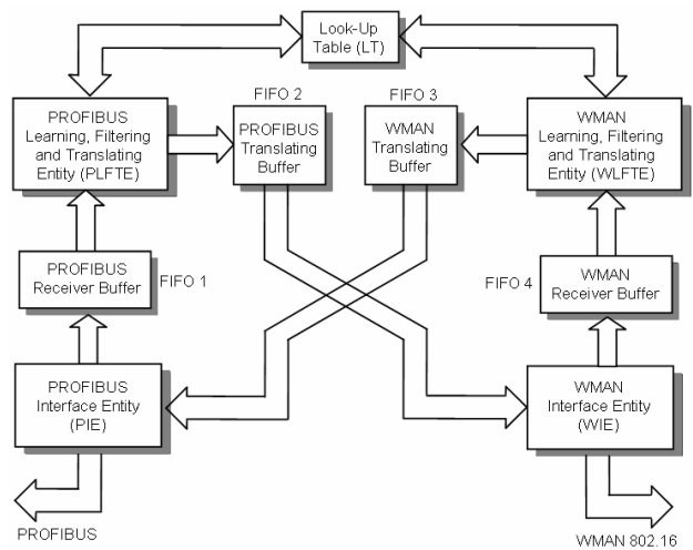
Fig. 5 Functional block diagram of the PROFIBUS/IEEE 802.16 WIU
