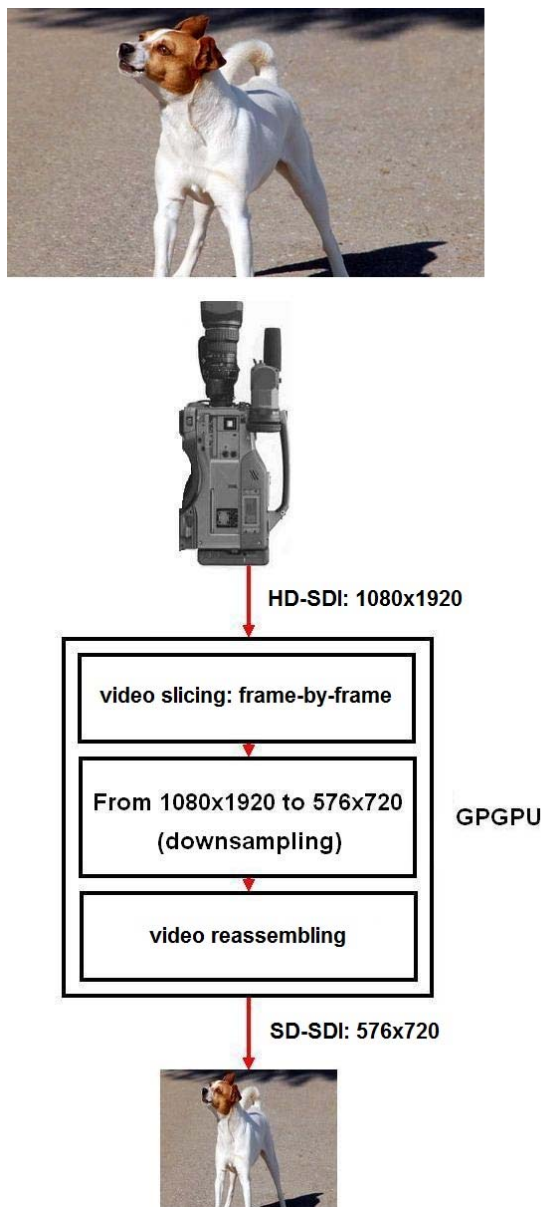
Fig.12: Encoder.
