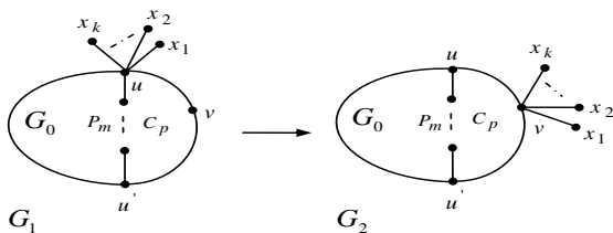
Fig. 2. Lemma2.2
