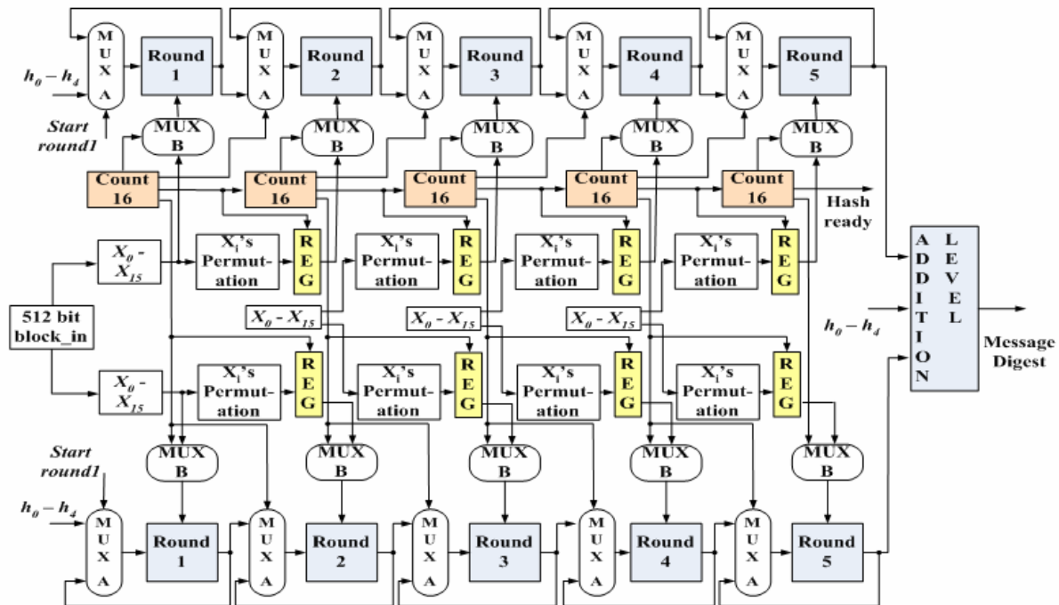
Fig. 2 Ripemd-160 Core
