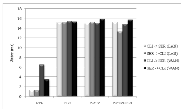
Fig. 14 GSM codec Jitter
