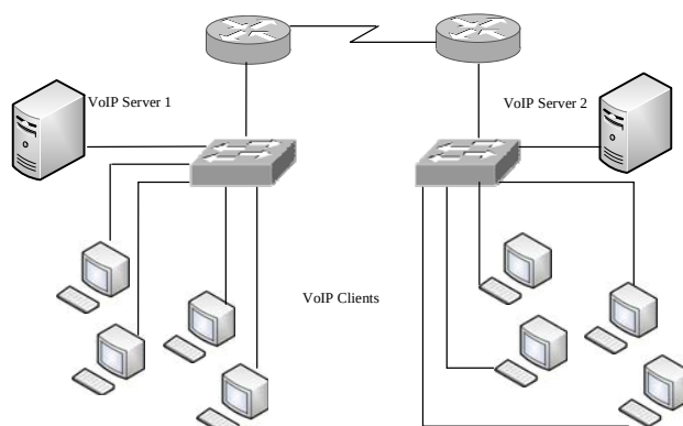
Fig. 3 WAN Scenario
