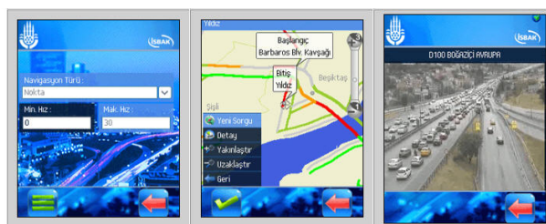
Fig. 1 IBBCepTrafik Screenshots [4].
