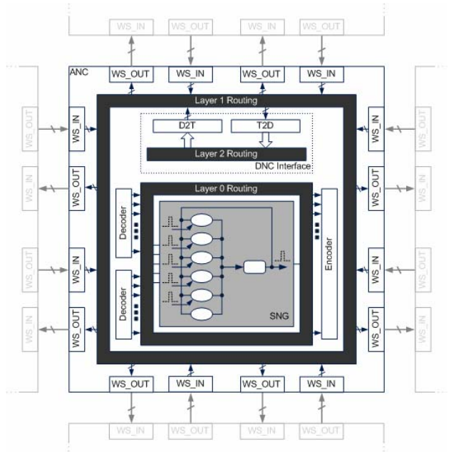
Fig. 1 ANC Schematic
