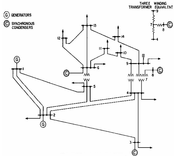
Fig. 7. IEEE 14-bus testing system.
